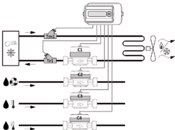
IMPIANTI A 2 TUBI - fig.1
