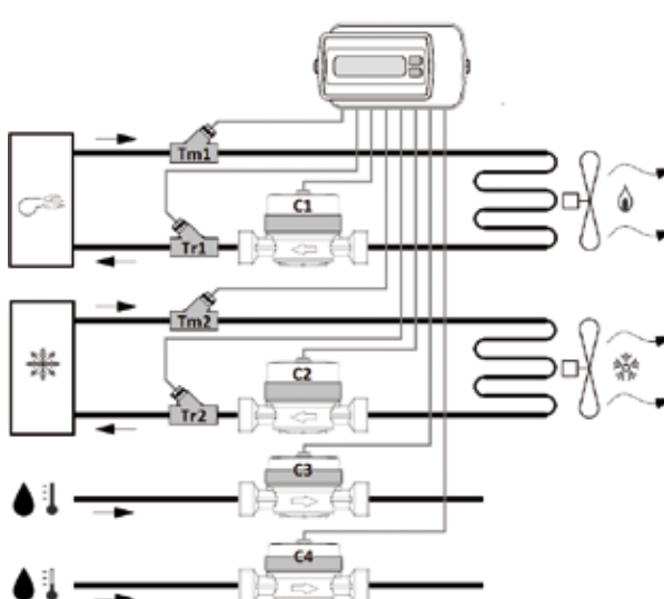
IMPIANTI A 4 TUBI - fig.2
