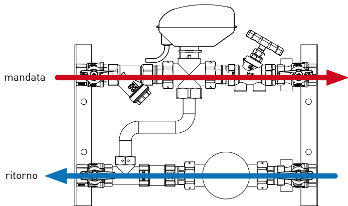
Valvola di zona aperta/passaggio dritto
