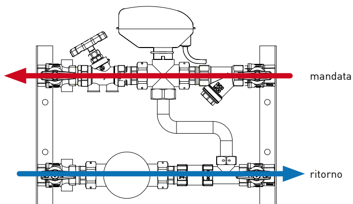
Valvola di zona aperta/passaggio dritto
