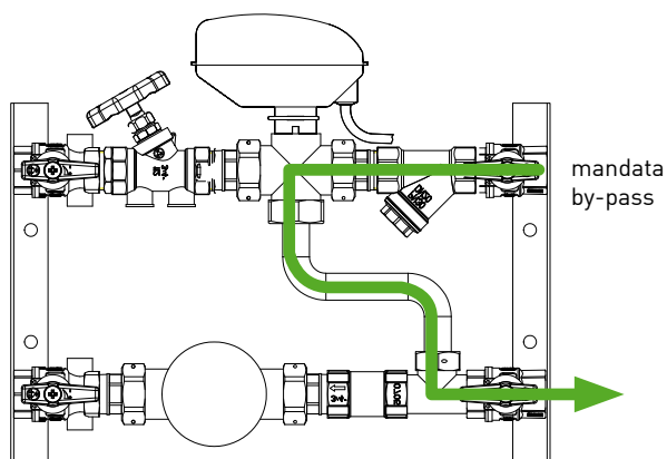
Valvola di zona chiusa/passaggio in by-pass
