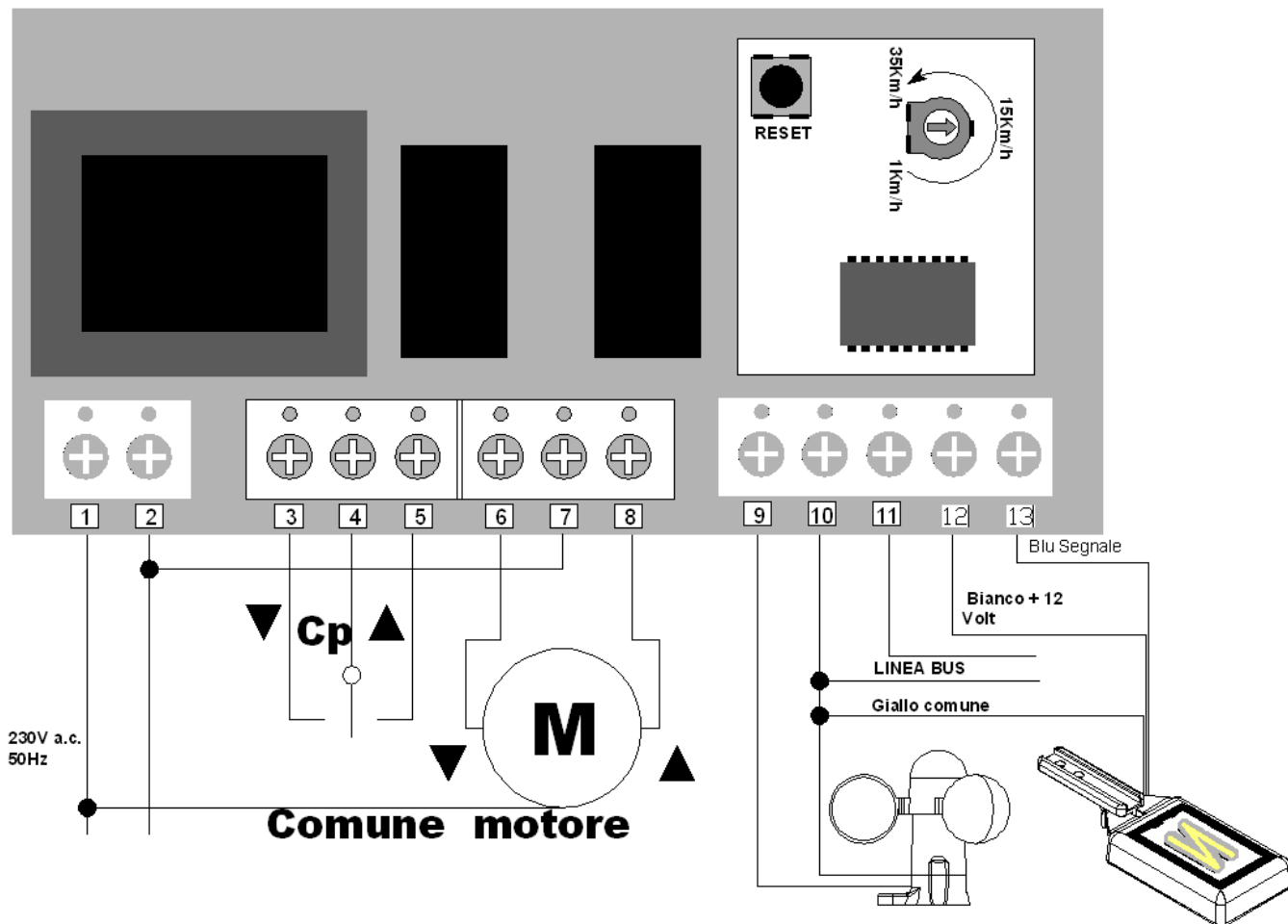
Schema di collegamento per 1 motore Schema 1
