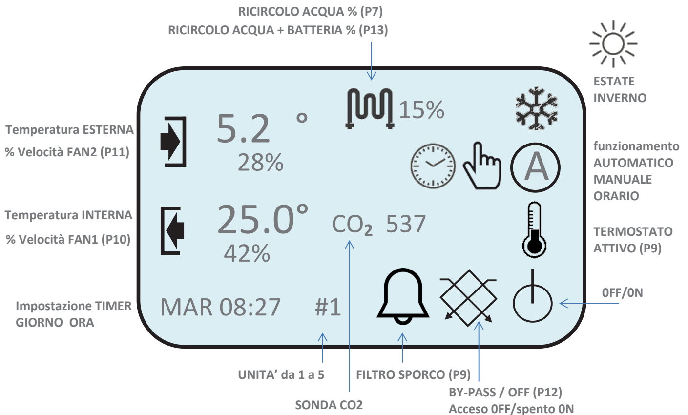
SCHEMATA DIMOSTRATIVA
