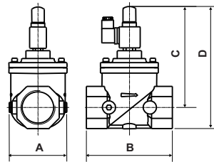
■ ZDEV...15 ÷ 50
