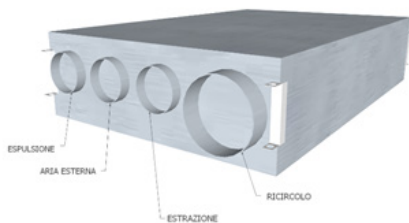
COLLEGAMENTI POSTERIORI
